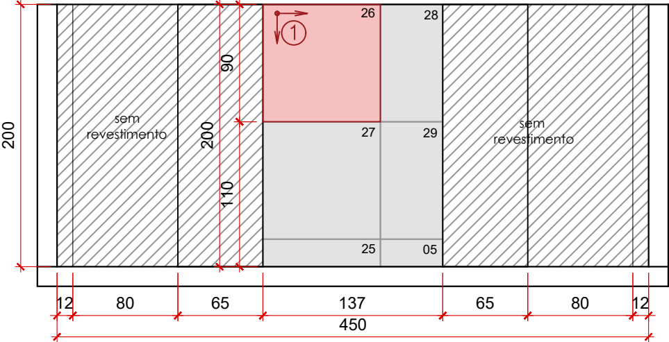
VISTA E - PAGINAÇÃO MURO esc.: 1/40
