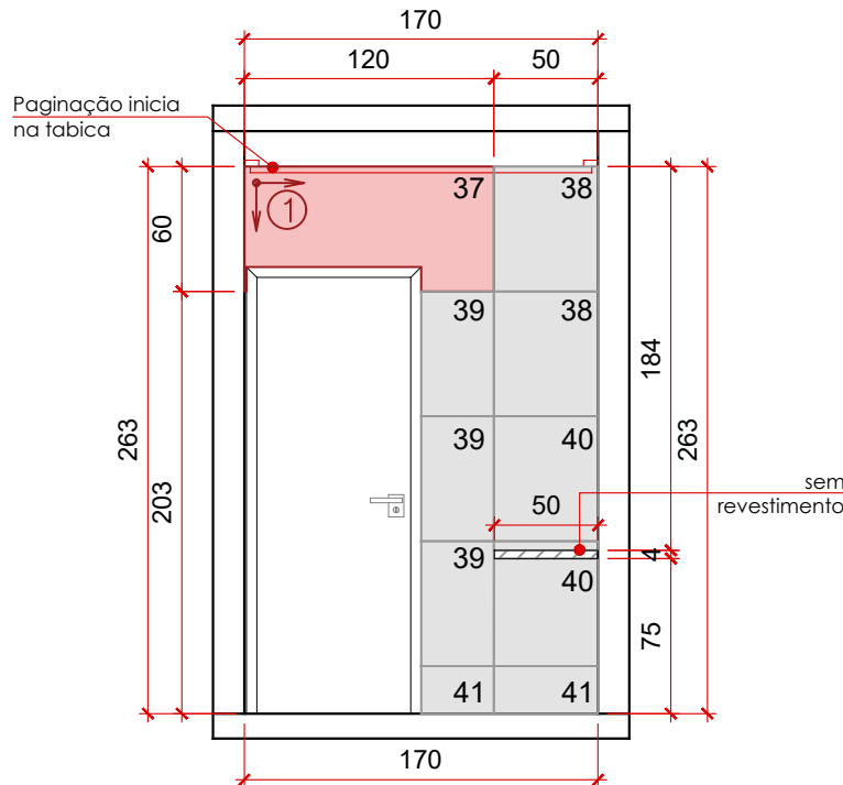
VISTA D - PAGINAÇÃO BANHO MASTER esc.: 1/40
