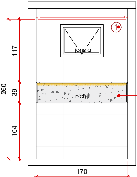
VISTA B - BANHO MASTER esc.: 1/40
