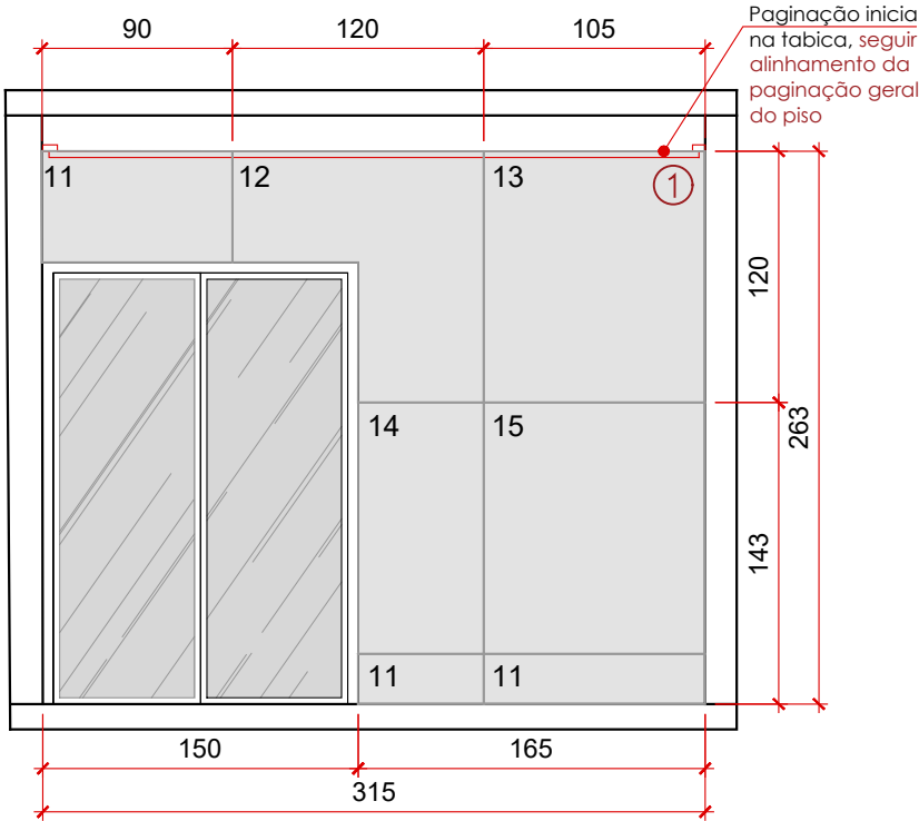
VISTA C - PAGINAÇÃO LAVANDERIA esc.: 1/40
