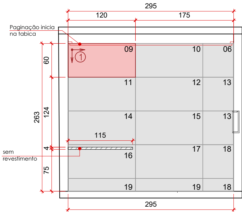
VISTA A - PAGINAÇÃO BANHO MASTER esc.: 1/40
