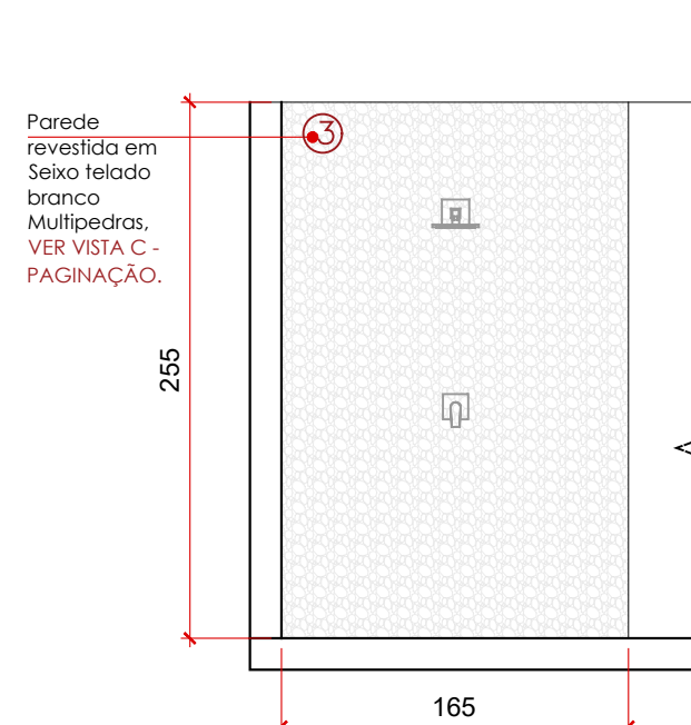
VISTA D - MURO esc.: 1/40
