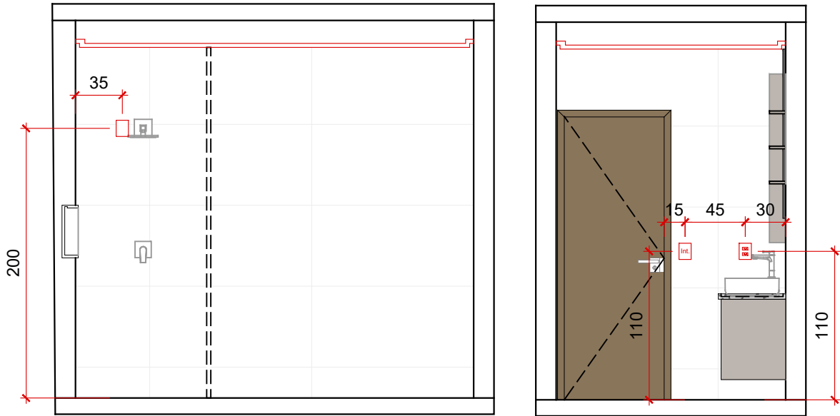
VISTA C - ELÉTRICO Banho master - esc.: 1/40
