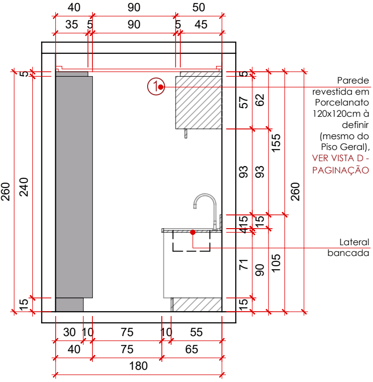
VISTA D - LAVANDERIA esc.: 1/40
