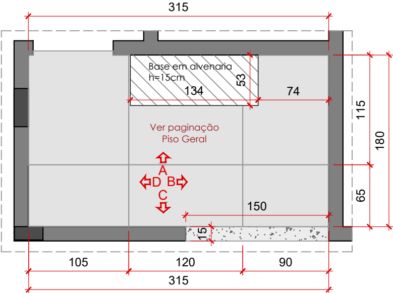
PLANTA BAIXA PAGINAÇÃO Lavanderia esc.: 1/40
