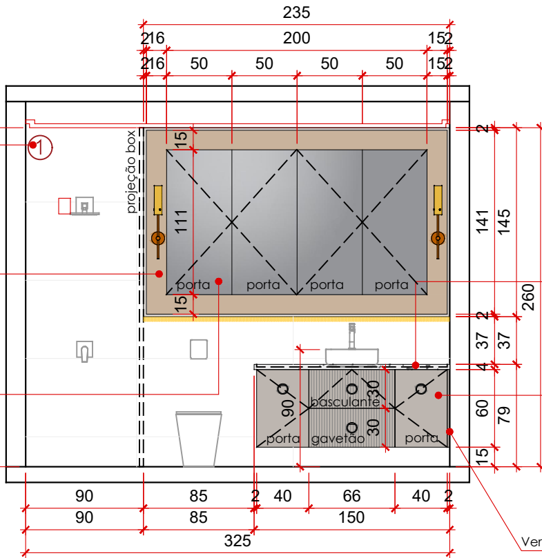
VISTA A - BANHO 02 esc.: 1/40
