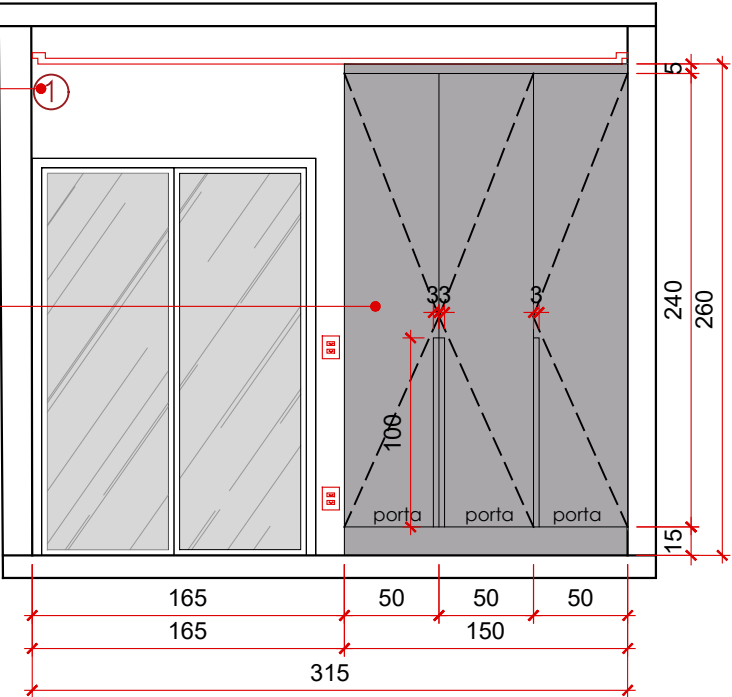
VISTA C - LAVANDERIA esc.: 1/40
