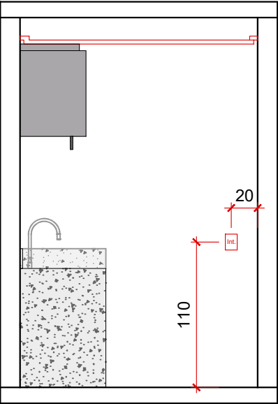
VISTA B - ELÉTRICO Lavanderia - esc.: 1/40
