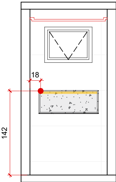
VISTA D - ELÉTRICO Banho 01 - esc.: 1/40
