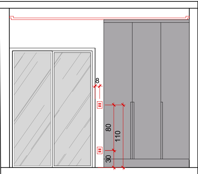
VISTA C - ELÉTRICO Lavanderia - esc.: 1/40
