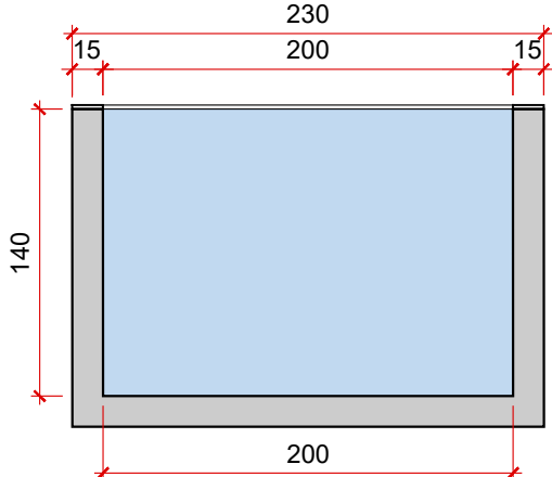
VISTA B - PISCINA esc.: 1/40
