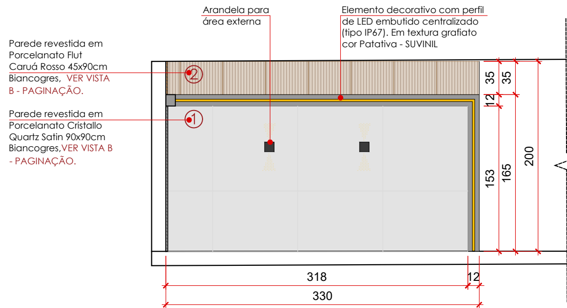
VISTA B - MURO esc.: 1/40
