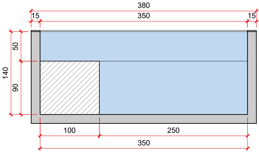
VISTA A - PISCINA esc.: 1/40
