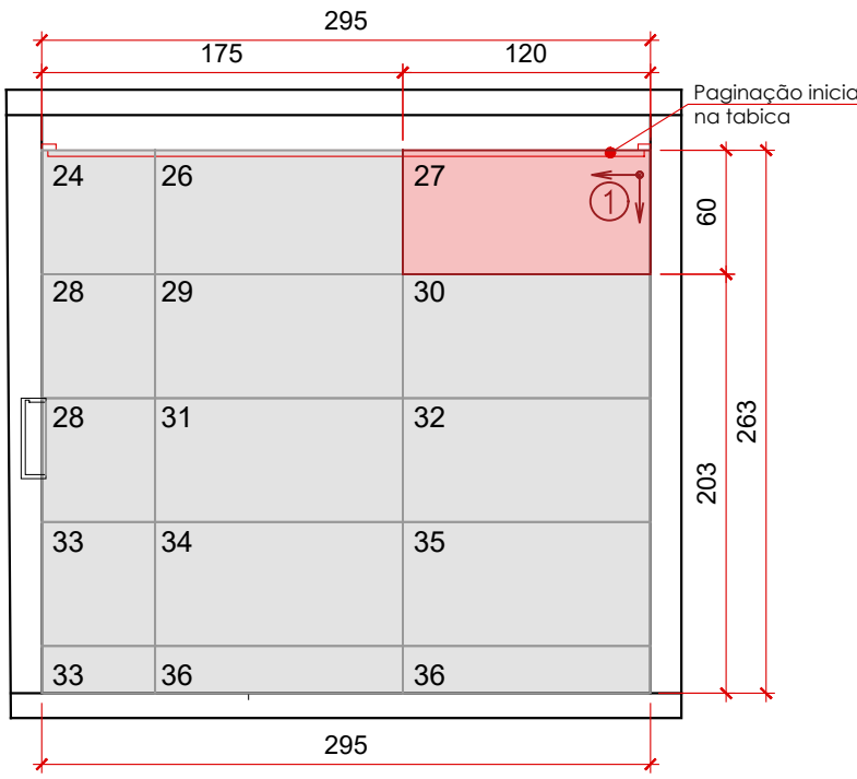
VISTA C - PAGINAÇÃO BANHO MASTER esc.: 1/40
