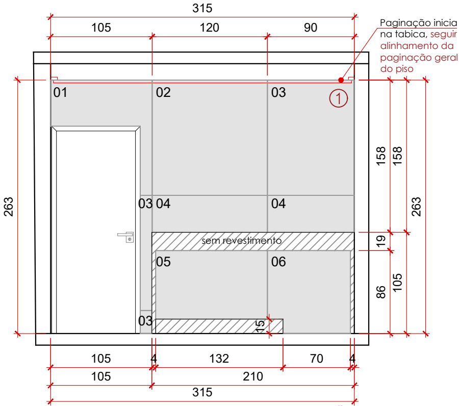
VISTA A - PAGINAÇÃO LAVANDERIA esc.: 1/40
