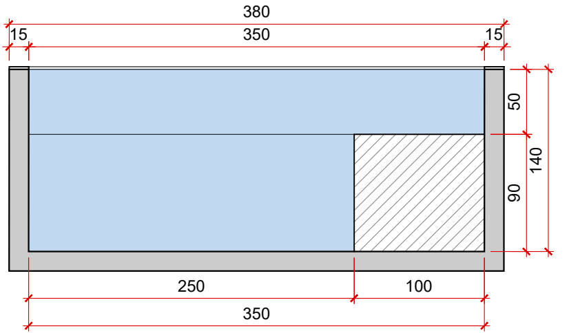
VISTA C - PISCINA esc.: 1/40
