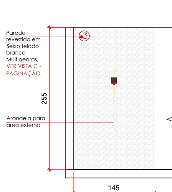
VISTA C - MURO esc.: 1/40
