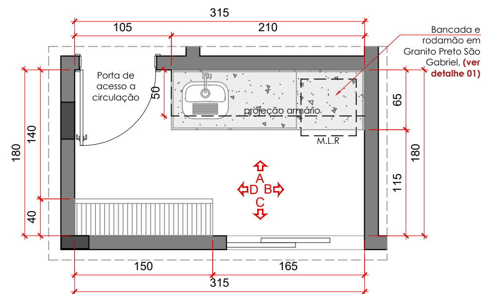
PLANTA BAIXA LAVANDERIA esc.: 1/40
