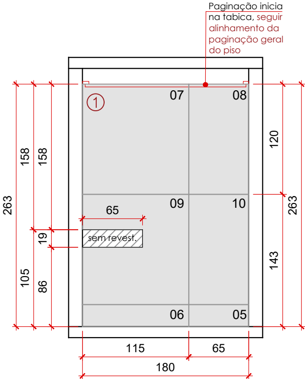
VISTA B - PAGINAÇÃO LAVANDERIA esc.: 1/40
