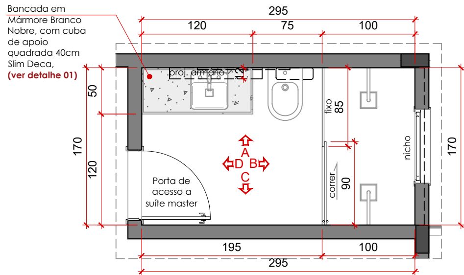
PLANTA BAIXA BANHO MASTER esc.: 1/40
