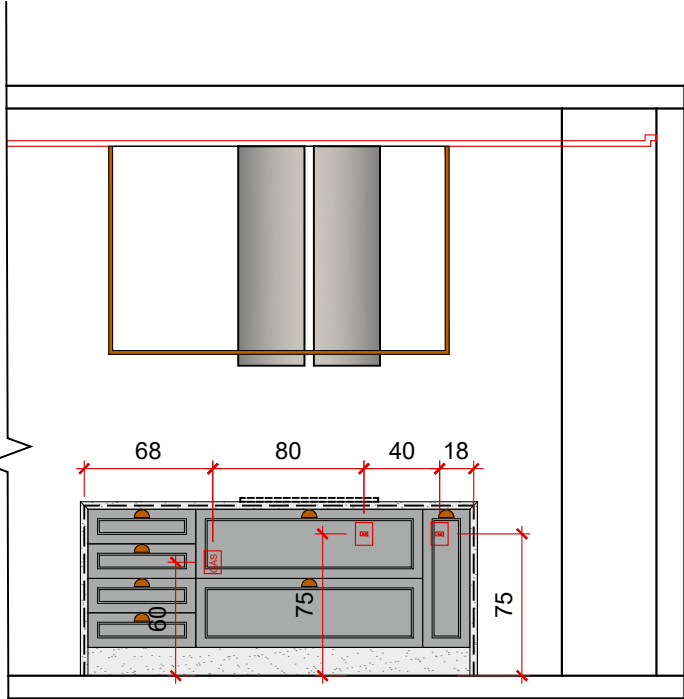
VISTA B - ELÉTRICO Varanda Gourmet - esc.: 1/40
