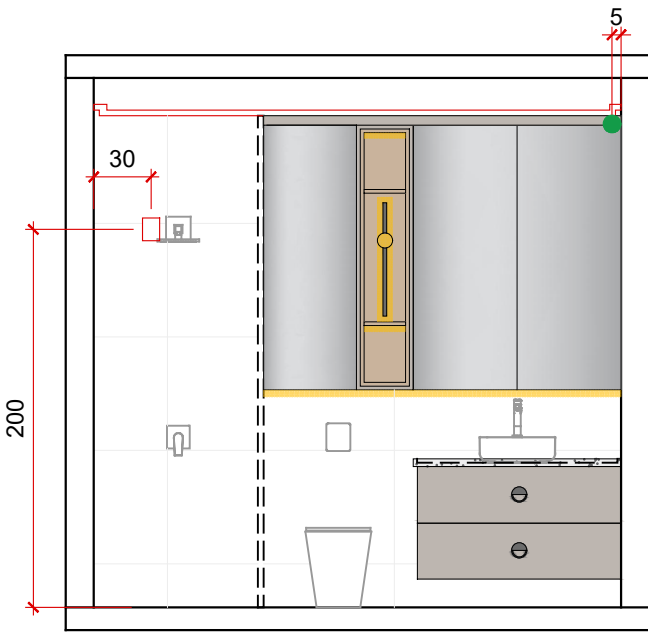
VISTA A - ELÉTRICO Banho 01 - esc.: 1/40
