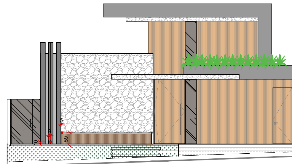
FACHADA FRONTAL esc.: 1/100
