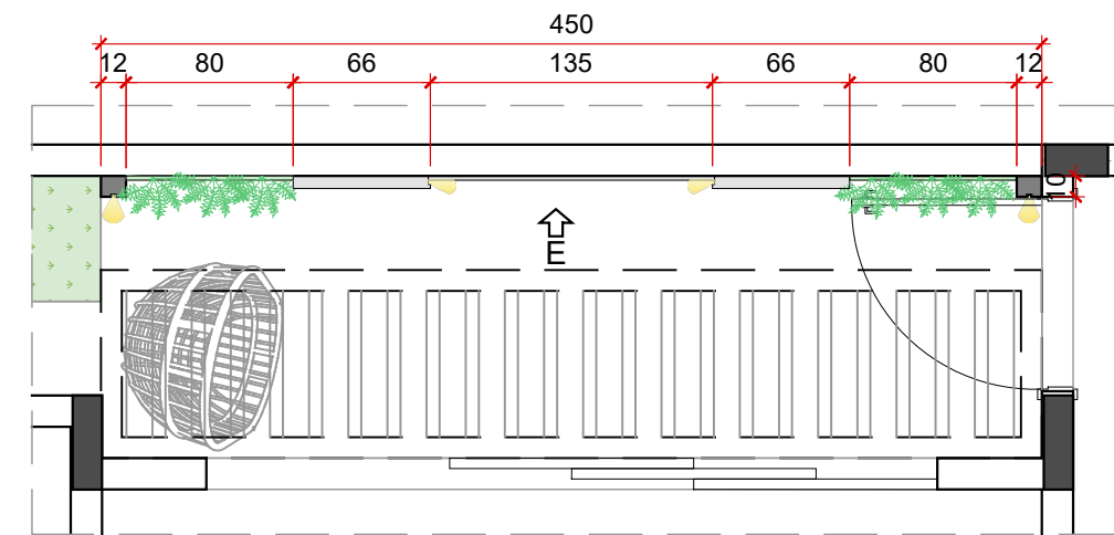
PLANTA MURO 2 esc.: 1/40
