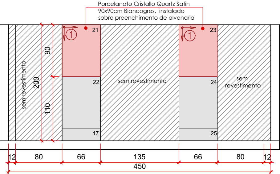
VISTA E' - PAGINAÇÃO MURO esc.: 1/40
