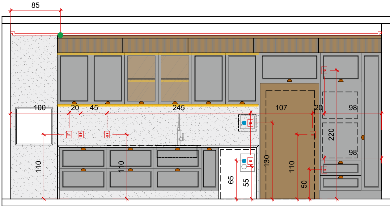
VISTA A - ELÉTRICO Varanda Gourmet - esc.: 1/40
