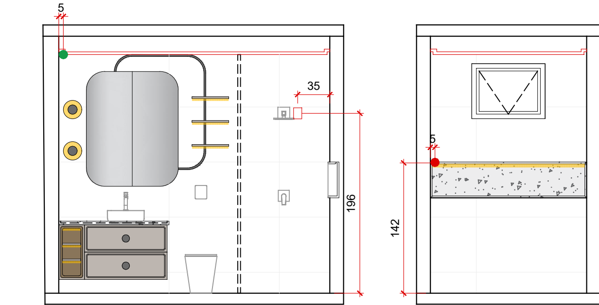
VISTA A - ELÉTRICO Banho master - esc.: 1/40
