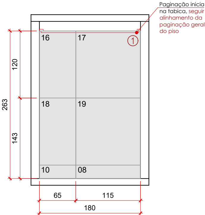
VISTA D - PAGINAÇÃO LAVANDERIA esc.: 1/40
