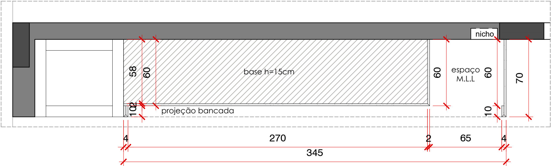
PLANTA BAIXA - SEM TAMPO
