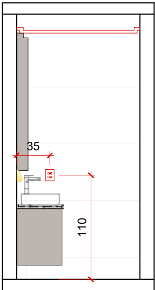
VISTA B - ELÉTRICO Banho 01 - esc.: 1/40
