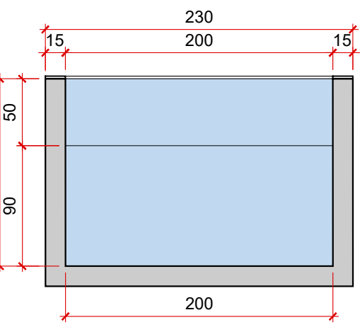
VISTA D - PISCINA esc.: 1/40
