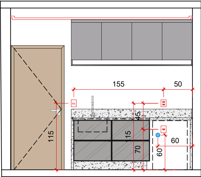
VISTA A - ELÉTRICO Lavanderia - esc.: 1/40
