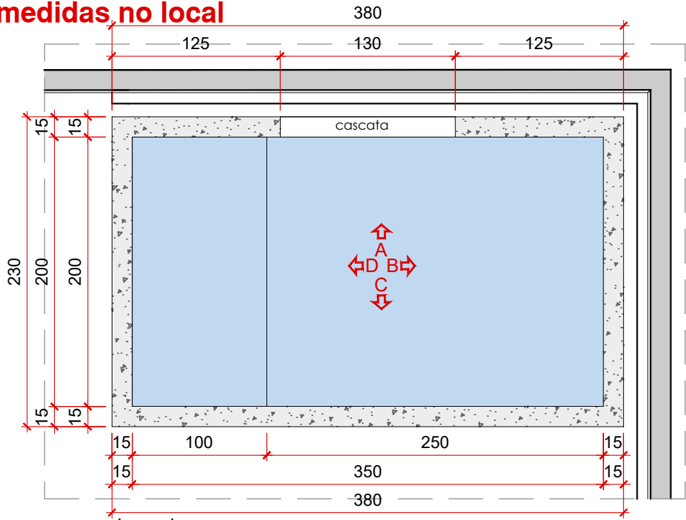
PLANTA BAIXA Piscina esc.: 1/40
