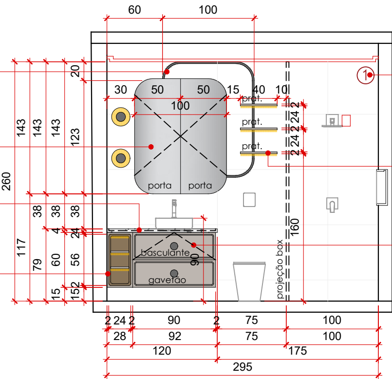
VISTA A - BANHO MASTER esc.: 1/40
