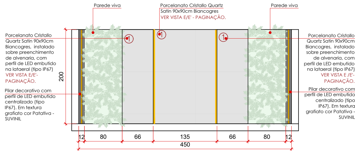
VISTA E - MURO esc.: 1/50
