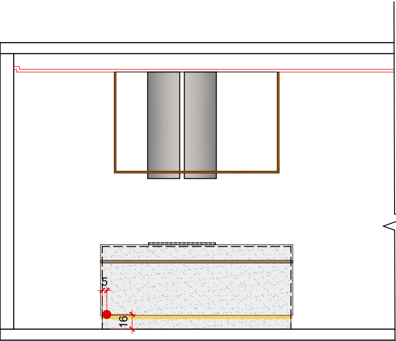
VISTA D - ELÉTRICO Varanda Gourmet - esc.: 1/40
