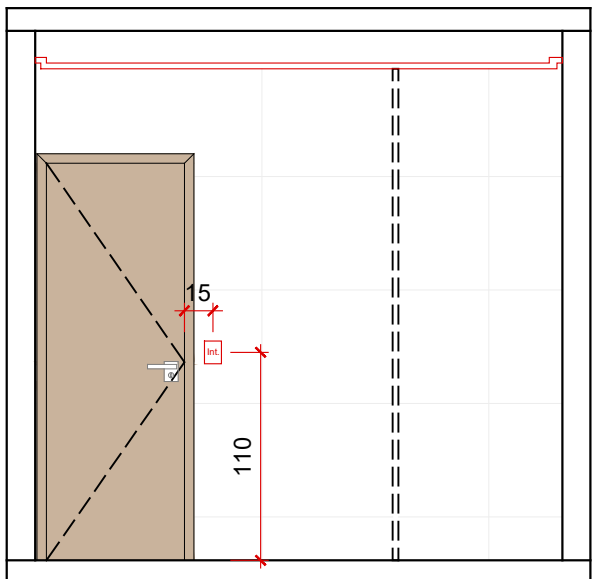
VISTA C - ELÉTRICO Banho 01 - esc.: 1/40
