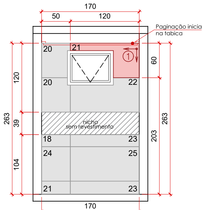
VISTA B - PAGINAÇÃO BANHO MASTER esc.: 1/40
